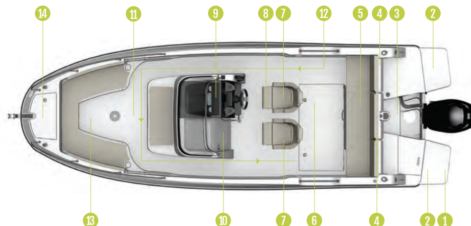
11 Cabine avec WC marin coulissant.
